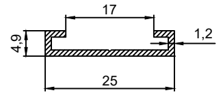
P.No 2020 0.125 Kg/m
