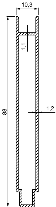
P.No 2016 0.612 Kg/m
