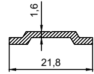
P.No 2019 0.110 Kg/m
