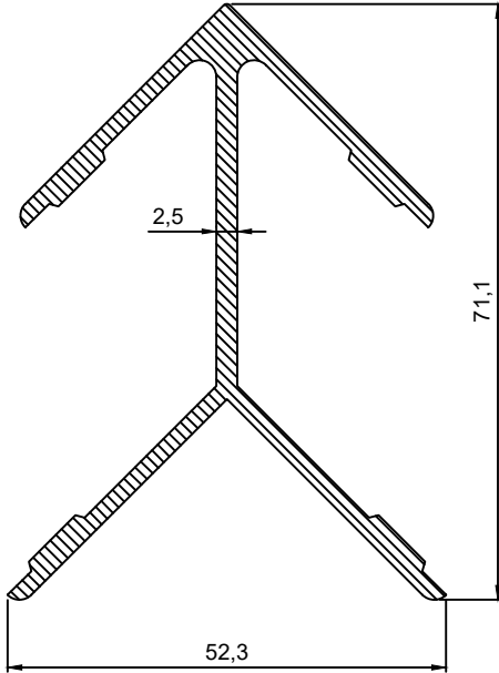
P.No 2021 1.160 Kg/m
