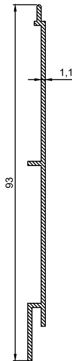
P.No 2017 0.320 Kg/m
