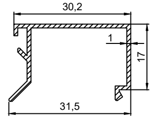
P.No 2015 0.214 Kg/m
