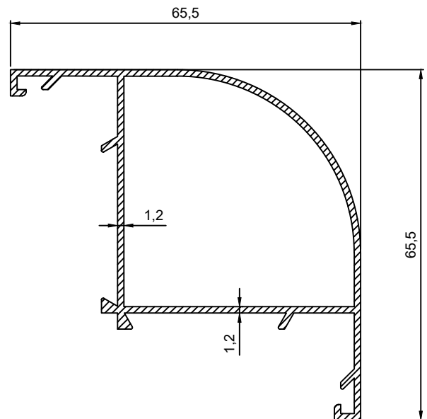
P.No 2013 0.772 Kg/m
