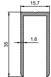
P.No 2024 0.365 Kg/m
