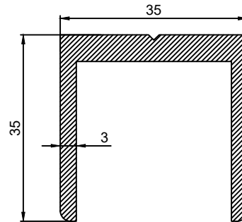
P.No 2023 0.951 Kg/m
