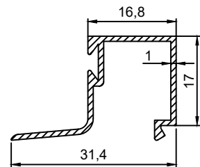
P.No 2014 0.213 Kg/m
