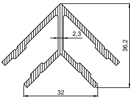
P.No 2022 0.821 Kg/m
