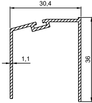
P.No 3204 0.309 Kg/m
