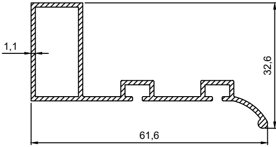
P.No 2853 0.450 Kg/m
