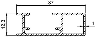
P.No 2849 0.279 Kg/m
