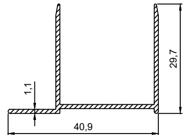
P.No 3203 0.287 Kg/m
