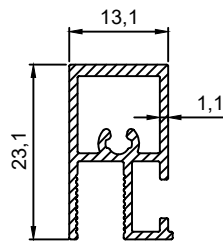
P.No 3201 0.257 Kg/m
