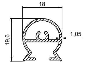
P.No 2848 0.241 Kg/m
