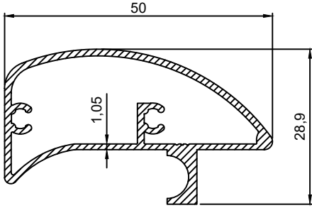
P.No 4560 0.566 Kg/m
