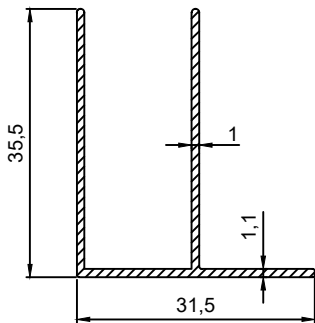
P.No 2860 0.279 Kg/m
