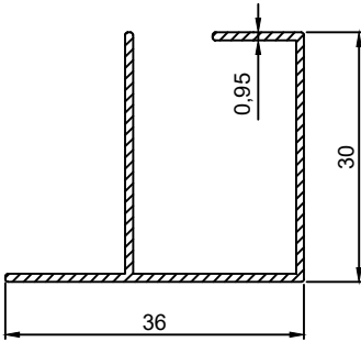
P.No 2881 0.268 Kg/m
