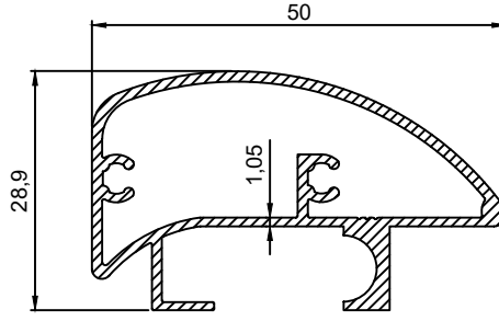
P.No 4563 0.612 Kg/m
