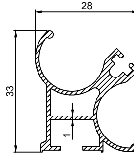
P.No 2858 0.406 Kg/m
