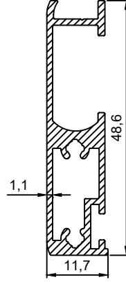
P.No 3205 0.455 Kg/m
