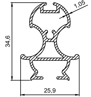
P.No 2852 0.431 Kg/m
