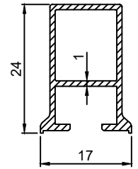
P.No 2859 0.228 Kg/m
