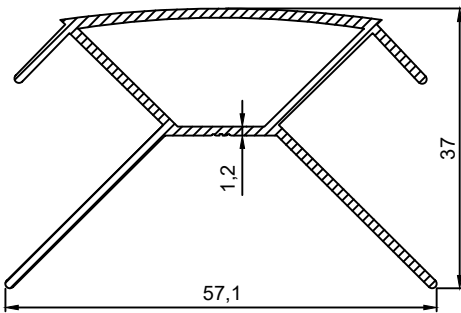
P.No 4564 0.566 Kg/m
