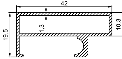
P.No 2882 0.451 Kg/m
