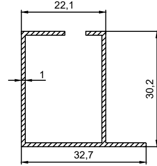
P.No 2887 0.286 Kg/m
