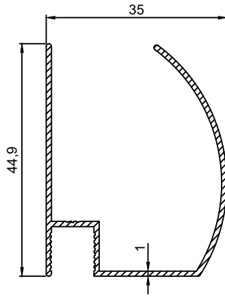
P.No 4561 0.352 Kg/m
