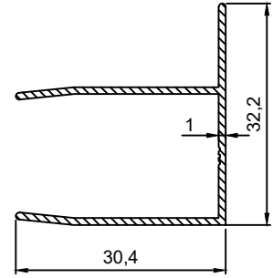
P.No 4565 0.244 Kg/m
