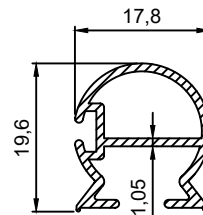
P.No 2847 0.225 Kg/m
