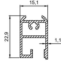
P.No 3638 0.285 Kg/m
