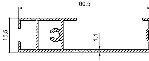
P.No 2851 0.455 Kg/m
