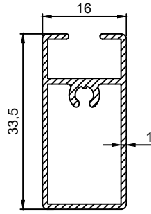
P.No 2855 0.314 Kg/m
