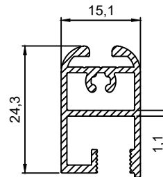
P.No 3202 0.316 Kg/m
