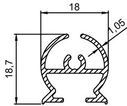
P.No 2846 0.230 Kg/m
