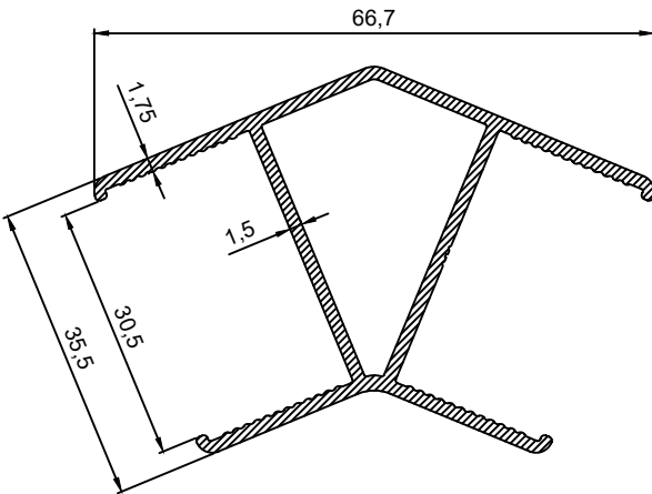
P.No 15059 0.767 Kg/m
