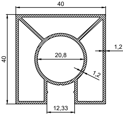
P.No 15037 0.851 Kg/m
