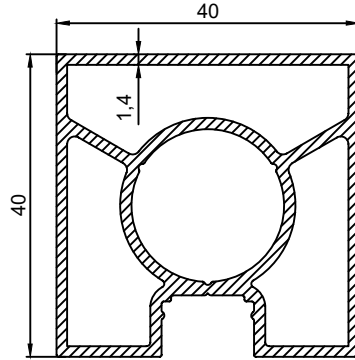
P.No 3505 0.991 Kg/m
