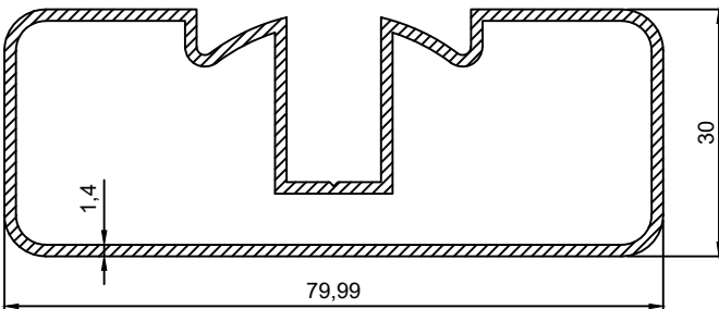
P.No 3511 0.980 Kg/m
