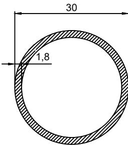
P.No 4288 0.431 Kg/m
