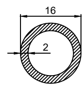
P.No 1003 0.240 Kg/m
