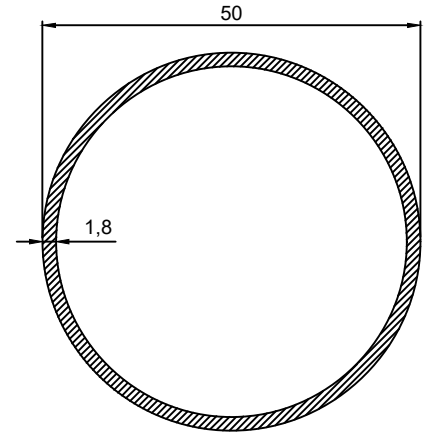
P.No 1013 0.740 Kg/m
