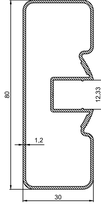
P.No 15047 0.832 Kg/m
