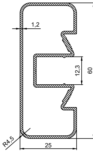
P.No 15050 0.686 Kg/m
