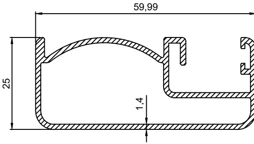
P.No 3509 0.756 Kg/m
