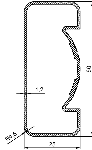
P.No 15049 0.593 Kg/m
