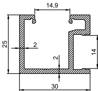
P.No 15044 0.515 Kg/m
