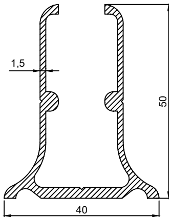
P.No 3513 0.767 Kg/m
