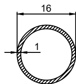
P.No 1001 0.130 Kg/m
