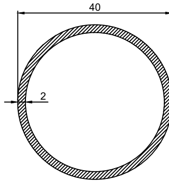
P.No 1010 0.645 Kg/m
