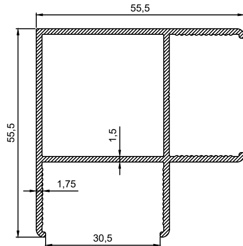
P.No 15060 0.902 Kg/m
