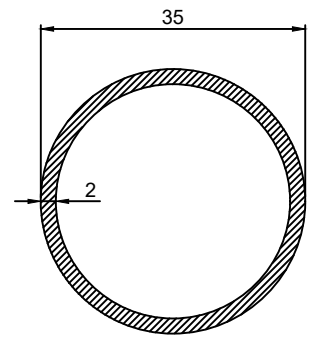
P.No 1008 0.560 Kg/m
