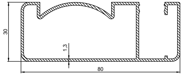
P.No 3516 0.905 Kg/m
