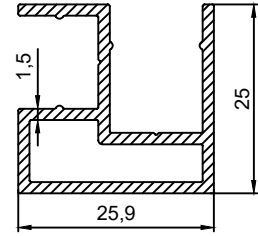
P.No 3848 0.448 Kg/m
