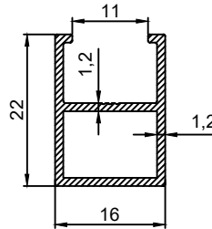
P.No 15040 0.239 Kg/m
