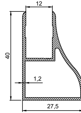
P.No 15052 0.461 Kg/m
