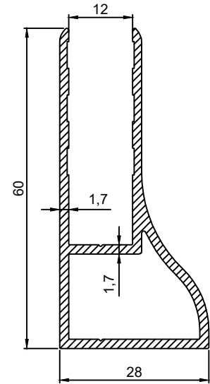
P.No 3849 0.750 Kg/m
