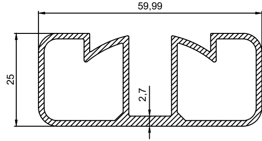
P.No 3508 0.873 Kg/m
