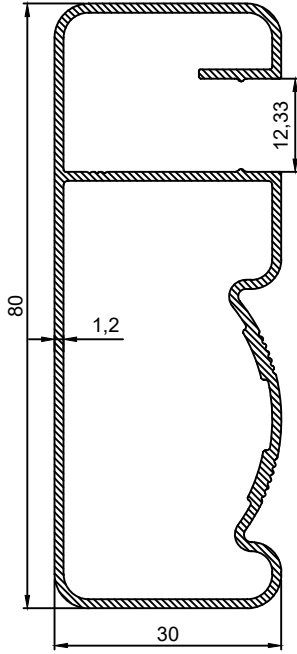
P.No 15046 0.816 Kg/m
