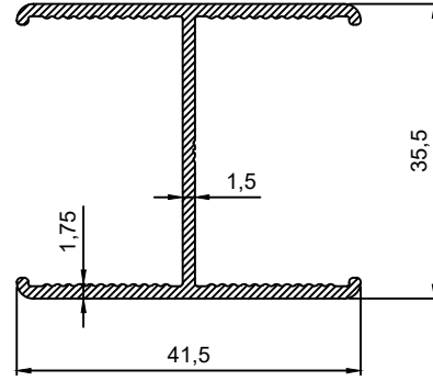
P.No 15058 0.493 Kg/m
