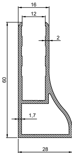
P.No 15054 0.813 Kg/m
