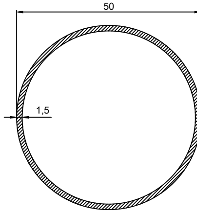
P.No 1012 0.620 Kg/m
