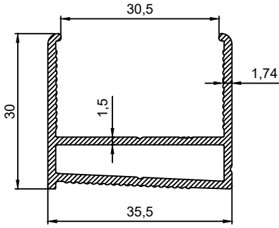
P.No 15057 0.526 Kg/m
