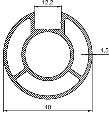
P.No 15034 0.854 Kg/m
