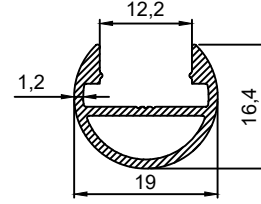
P.No 15035 0.217 Kg/m
