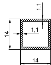
P.No 15042 0.153 Kg/m
