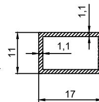
P.No 15041 0.153 Kg/m
