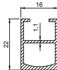
P.No 3512 0.268 Kg/m
