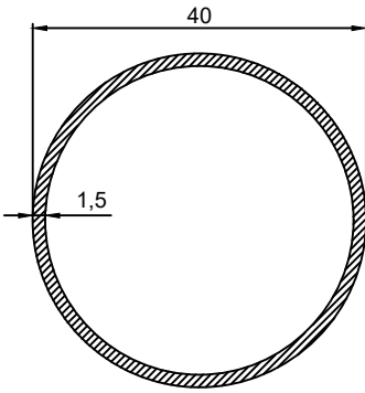
P.No 1009 0.490 Kg/m
