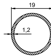
P.No 1004 0.181 Kg/m
