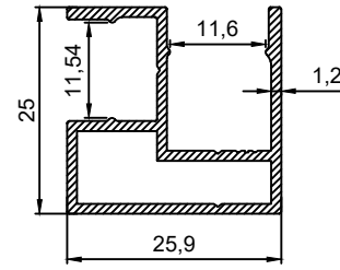
P.No 15039 0.374 Kg/m
