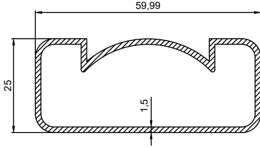
P.No 3507 0.710 Kg/m
