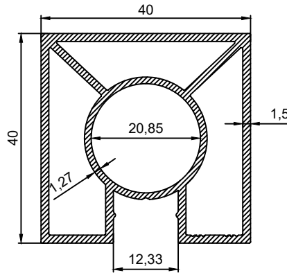
P.No 15038 0.997 Kg/m
