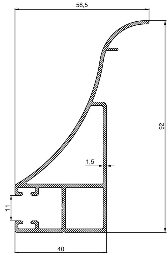
P.No 15051 1.111 Kg/m
