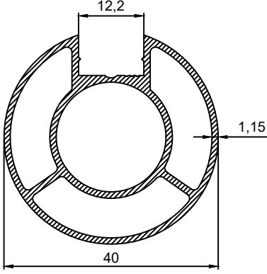
P.No 15033 0.691 Kg/m
