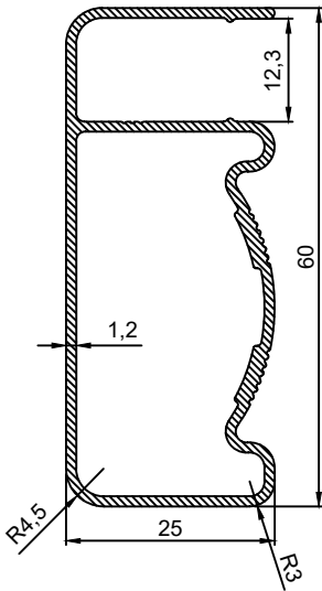
P.No 15048 0.604 Kg/m
