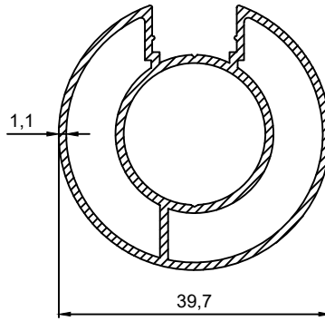
P.No 3502 0.624 Kg/m
