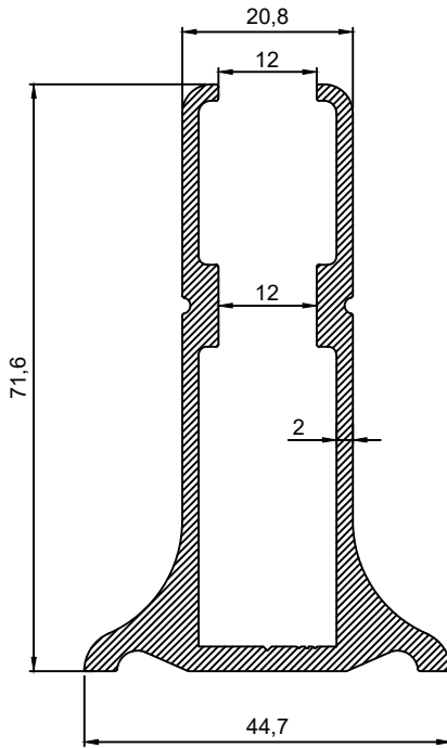
P.No 15053 1.439 Kg/m
