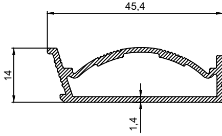
P.No 15055 0.439 Kg/m
