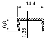
P.No 15045 0.076 Kg/m
