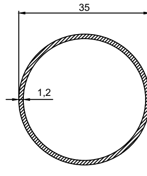
P.No 1026 0.345 Kg/m
