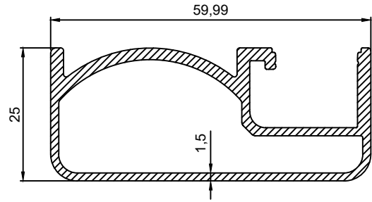
P.No 3510 0.911 Kg/m
