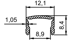
P.No 15036 0.076 Kg/m
