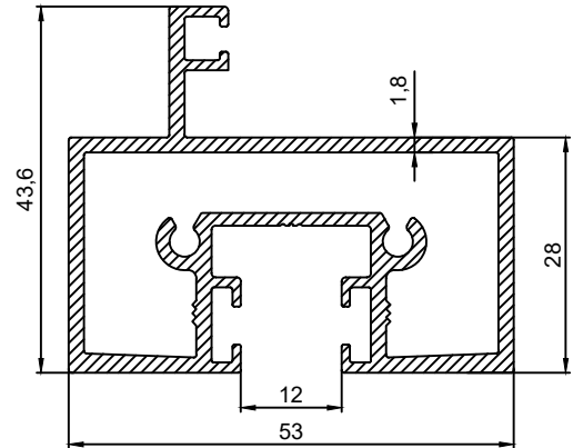
P.No 15070 0.425 Kg/m
