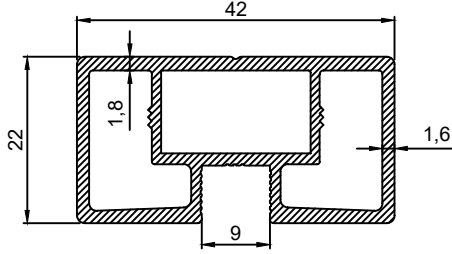
P.No 15067 0.737 Kg/m
