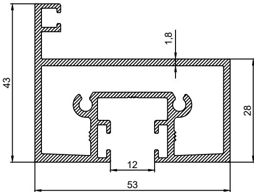
P.No 15071 1.182 Kg/m
