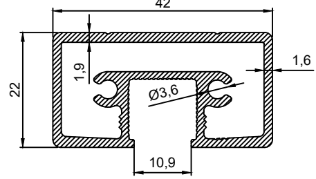
P.No 15068 0.783 Kg/m
