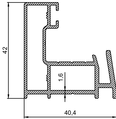
P.No 15069 0.764 Kg/m
