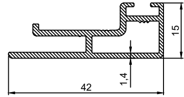
P.No 15070 0.425 Kg/m
